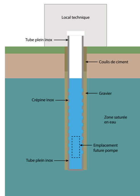
Schéma de principe d'un forage
