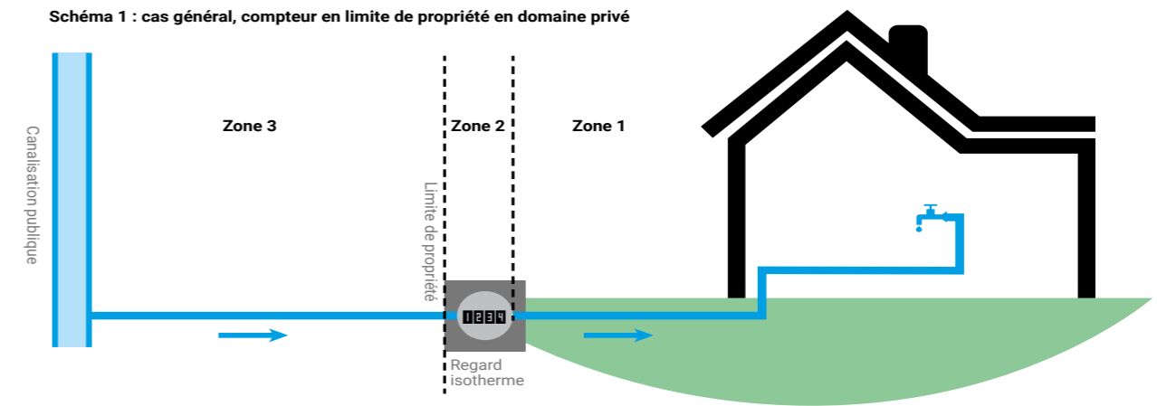
Schéma 1 : cas général, compteur en limite de propriété en domaine privé
