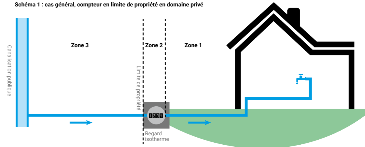
Schéma 1 : cas général, compteur en limite de propriété en domaine privé
